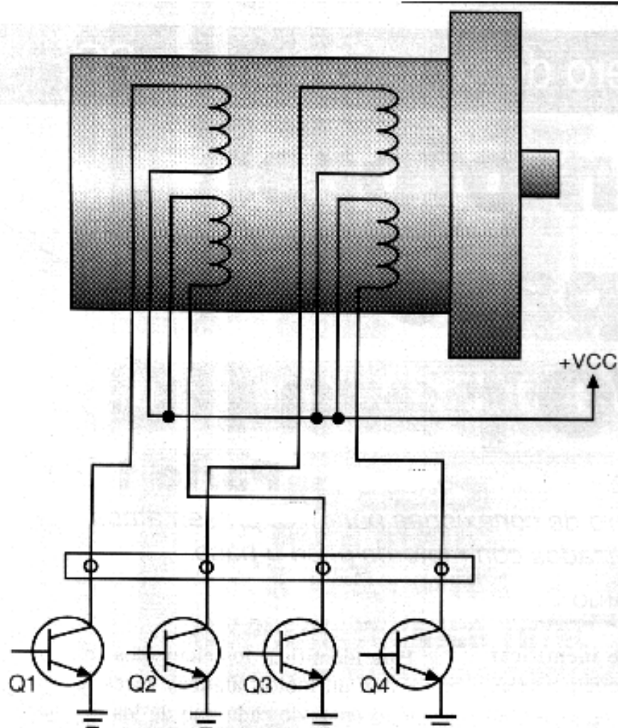
Figura 2. Conexión básica
